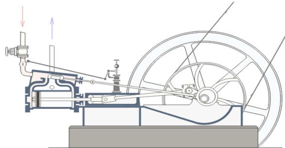
Maszyna parowa Źródło: Panther, CC BY-SA 3.0.
