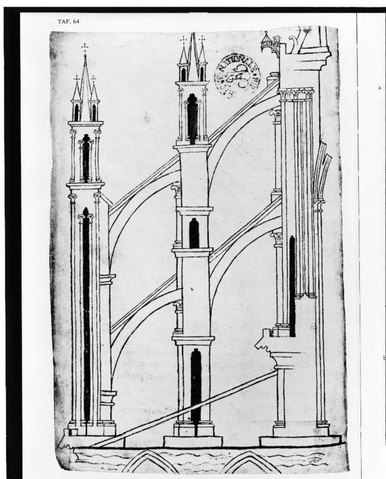
Villard de Honnecourt, przekrój katedry gotyckiej, rok i miejsce nieznane, cdn.loc.gov , CC BY 3.0
