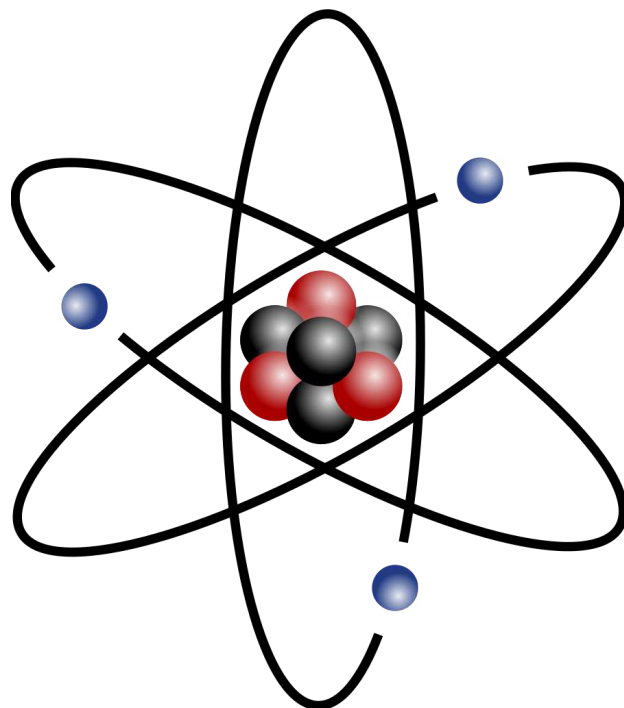
Współczesny model budowy atomu.
