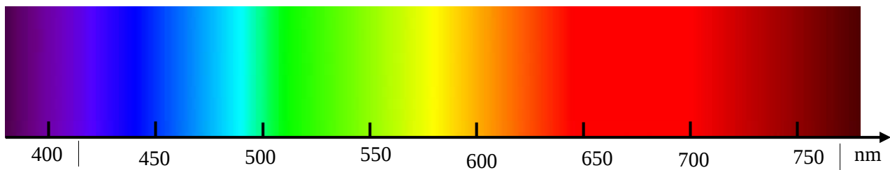
Rys. 1. Widmo światła widzialnego.
