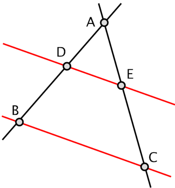
Ilustracja twierdzenia Talesa
