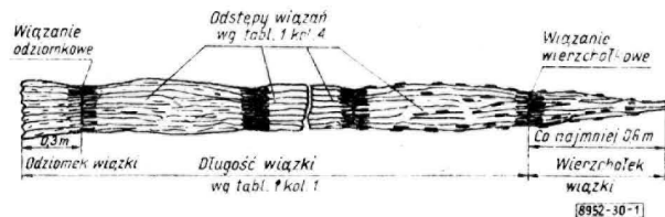
Rys. 1. Wiązka faszyny
